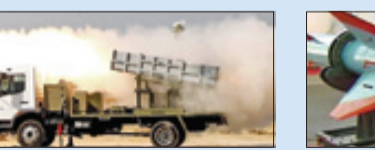
شلیک نصر از پرتابگر ساحلی
