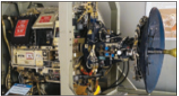
آنتن و اجزای دیگر رادار APQ-120 جنگنده اف ۴ فانتوم
