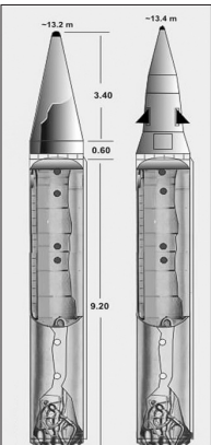
❧ مقایسه موشک خرمشهر (۱ و ۲) توسط یک تحلیلگر خارجی
